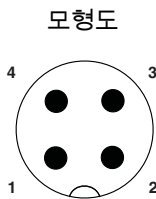
핀 할당 M12 플러그, 4핀, A-코드, 플러그 측면
