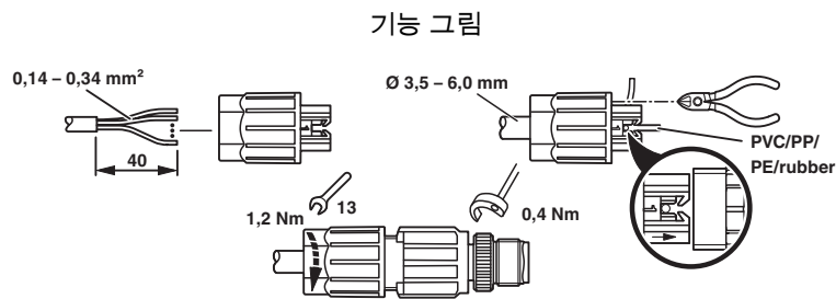
플러그, M12 x 1, 직선, 차폐
