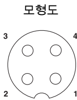
핀 할당 M12 소켓, 4핀, A-코드, 암 측면
