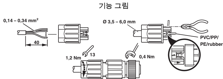
M12 x 1 암 커넥터, 직선
